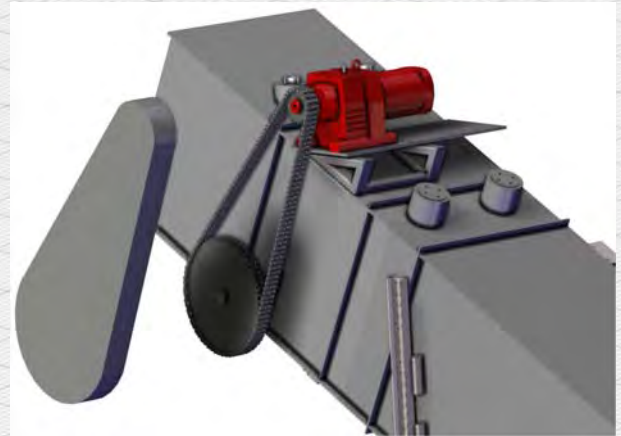
Antriebsstation
